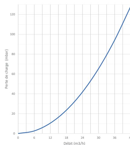
Pertes de charge à débit maximal : 122 mbar
