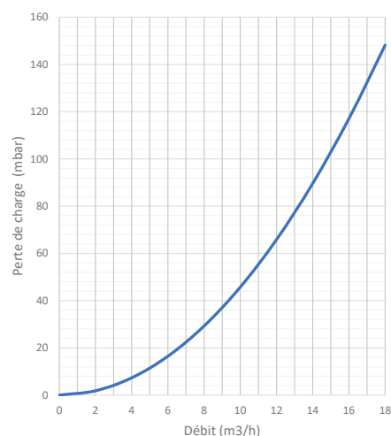
Pertes de charge à débit maximal : 140 mbar
