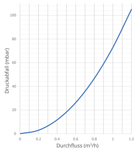
Druckabfall bei Maximalfluss: 105 mbar
